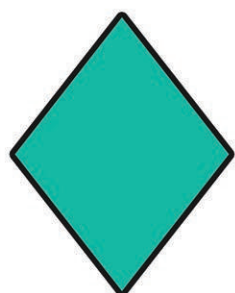
rhombus
