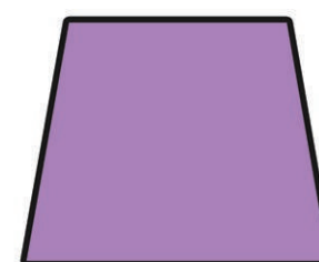
trapezium
